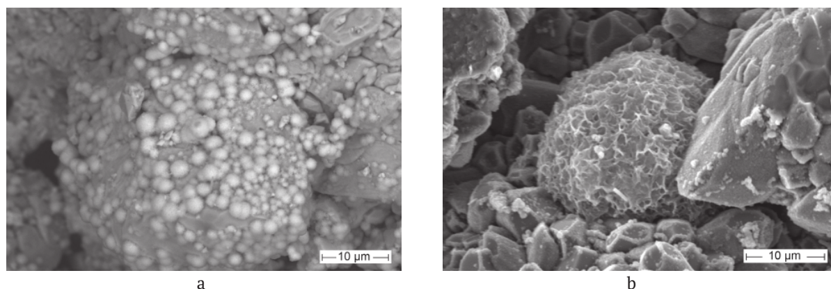
Рис. 14. Скопления коккоидных фоссилизированных бактерий (a — скол, режим BSE; b — скол, режим SE)
