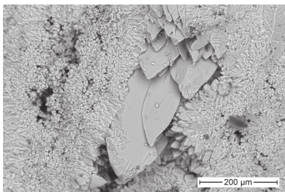
Рис. 6. Скаленоэдрические кристаллы кальцита (скол, режим BSE)
