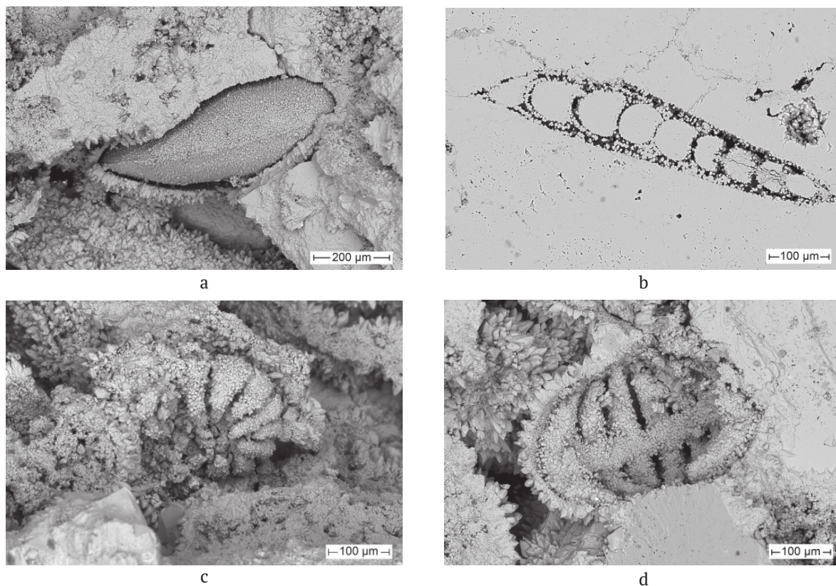
Рис. 4. Микрофоссилии (а — остракода (?); b–d — фораминиферы). а, с, d — сколы, b — аншлиф (режим BSE)
