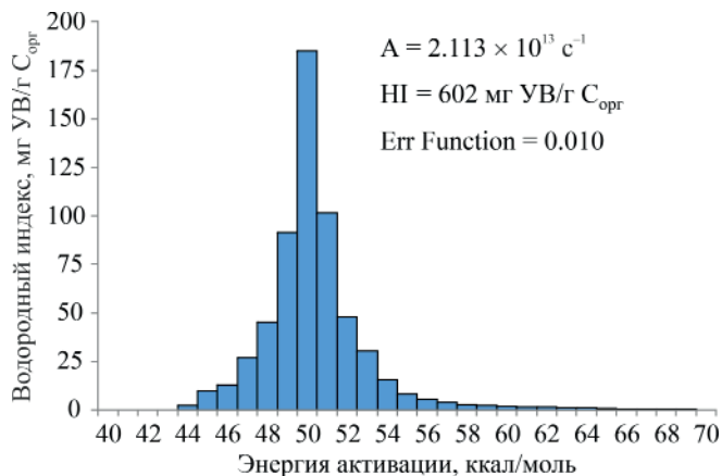
Рис. 1. Гистограмма распределения HI по E a исходного для автоклавного эксперимента образца доманикового сланца обнажения Чуть-Устье. Получено при выполнении работ по гранту РНФ 23-27-00139 (2023–2024)
